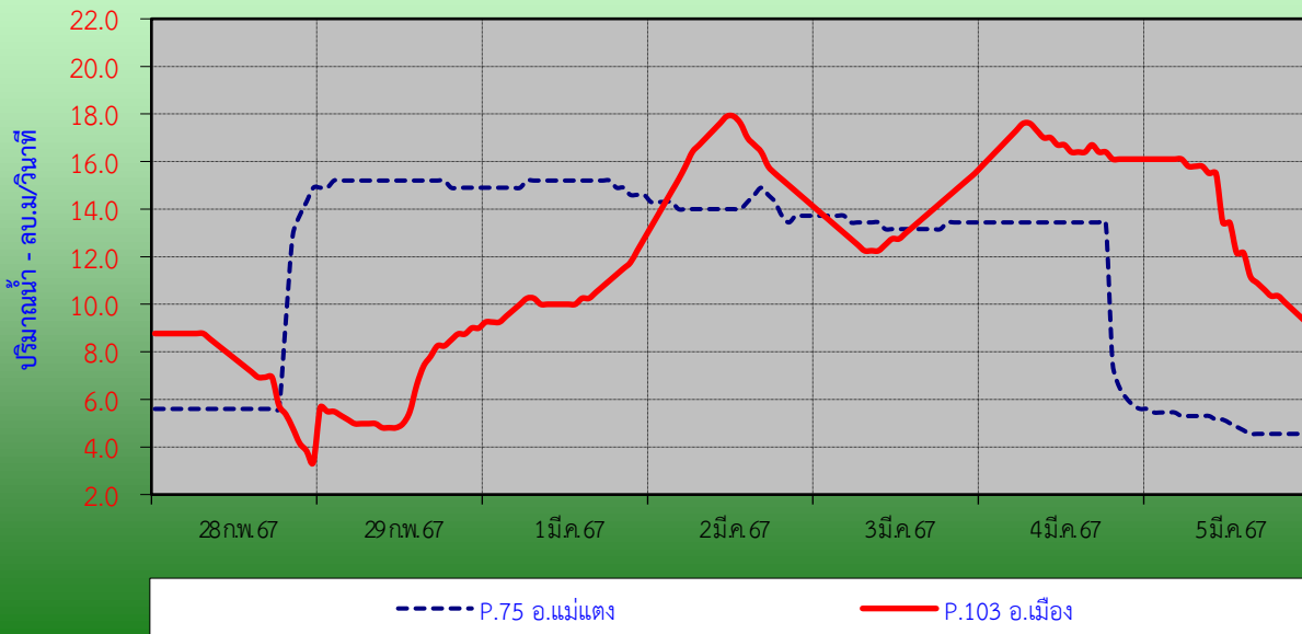
กราฟแสดงปริมาณน้ำปิ้งรายชั่วโมงรอบวันที่ 9/2567 ที่สถานีแม่ น้ำปิ้ง ( P.75) บ้านซ้อแล อ.แม่แตง และที่สถานีแม่ น้ำปิ้ง ( P.103) บ้านป่าซ้อยใต้ อ.เมือง จ.เชียงใหม่
